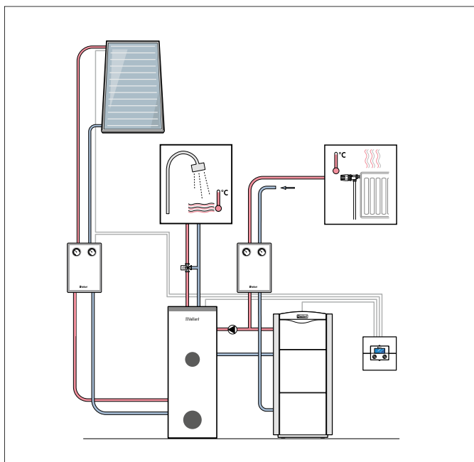
thermisch zonnepaneel auroTHERM, zonneboiler auroSTOR en condensatievloerketel op gas ecoVIT exclusiv
