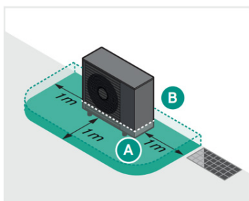
aroTHERM plus/8.1 met Flexible Space Function uitgeschakeld
