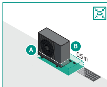
aroTHERM plus/8.1 met Flexible Space Function ingeschakeld
