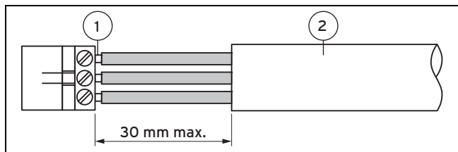
1 Aansluitdraden 2 Isolatie
