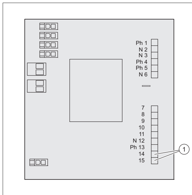
1 Uitgang 14-15
