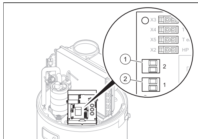
1 Aansluitklem 2 2 Aansluitklem 1
