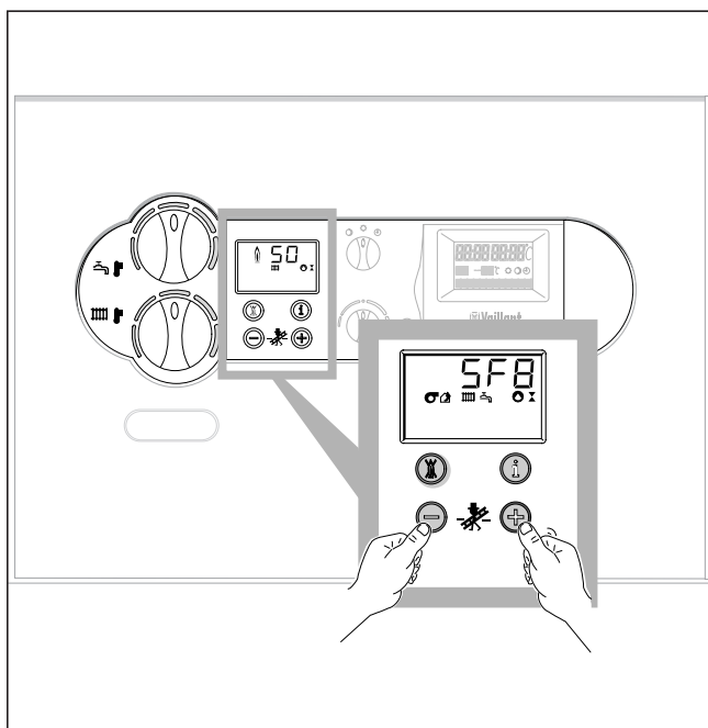
Afb. 6.1 Schoorsteenvegerbedrijf activeren
