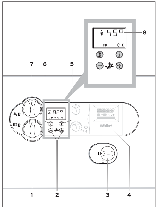
Afb. 4.2 Bedieningselementen
