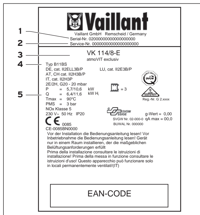
Afb. 2.1 Typeplaatje (voorbeeld)
