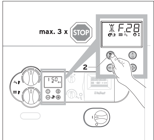
Afb. 5.1 Ontstoring
