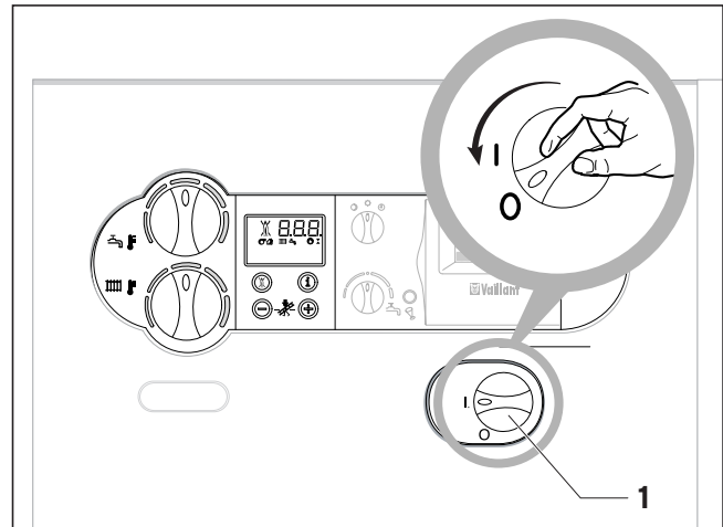
Afb. 4.3 Ketel in- en uitschakelen
