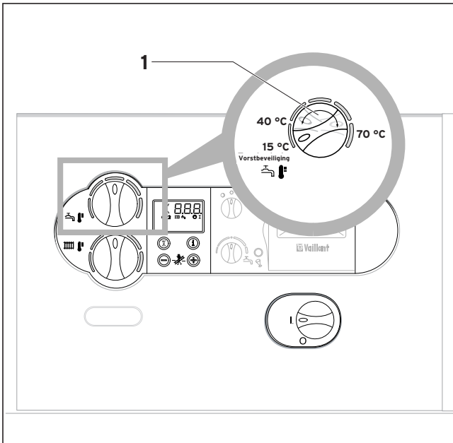
Afb. 4.5 Warmwaterbereiding (alleen bij aangesloten warmwaterreservoir)
