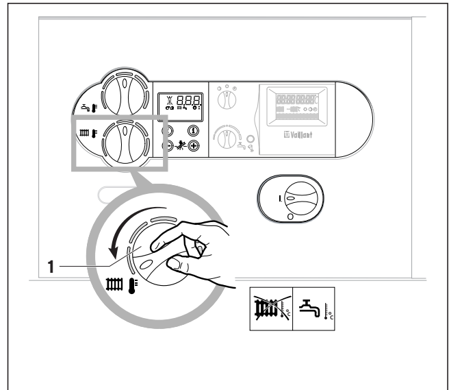
Afb. 4.8 Verwarmingsbedrijf uitschakelen (zomerbedrijf)
