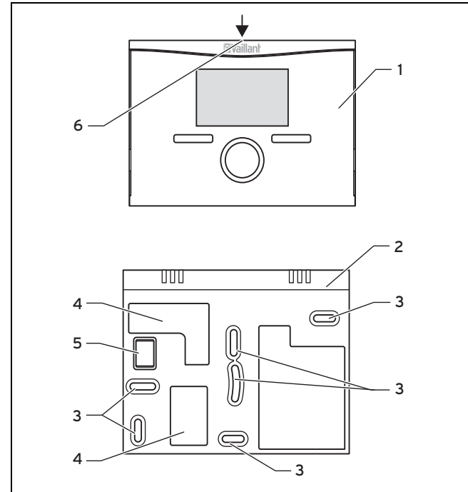
1 Thermostaat 2 Wandsokkel 3 Bevestigingsopeningen
