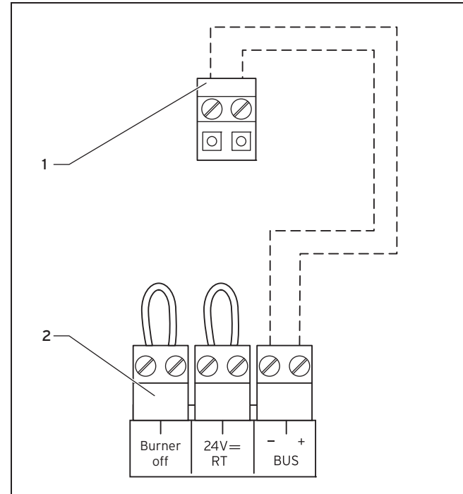
1 Klemmenlijst draadloze 2 Klemmenlijst CV-ketel ontvangereenheid
