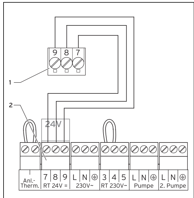
Afbeelding 5.1: Thermostaat aansluiten
