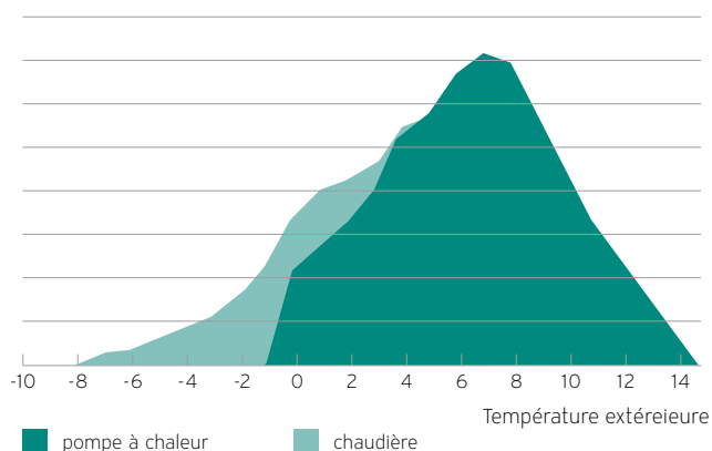
Demande de chaleur par pompe à chaleur et chaudière
