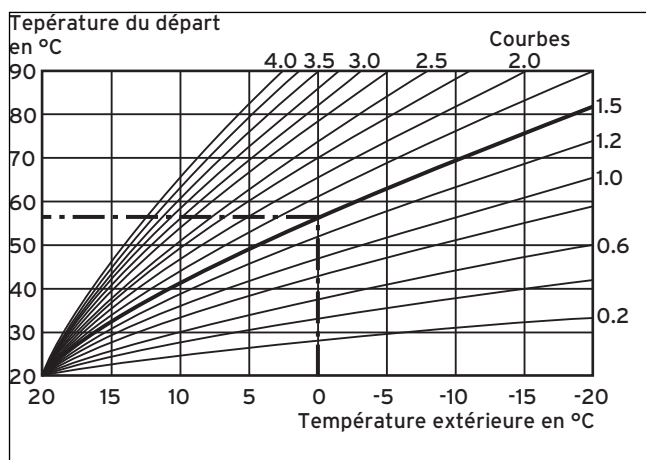
Fig. 3.3 Diagramme avec courbes de chauffage
