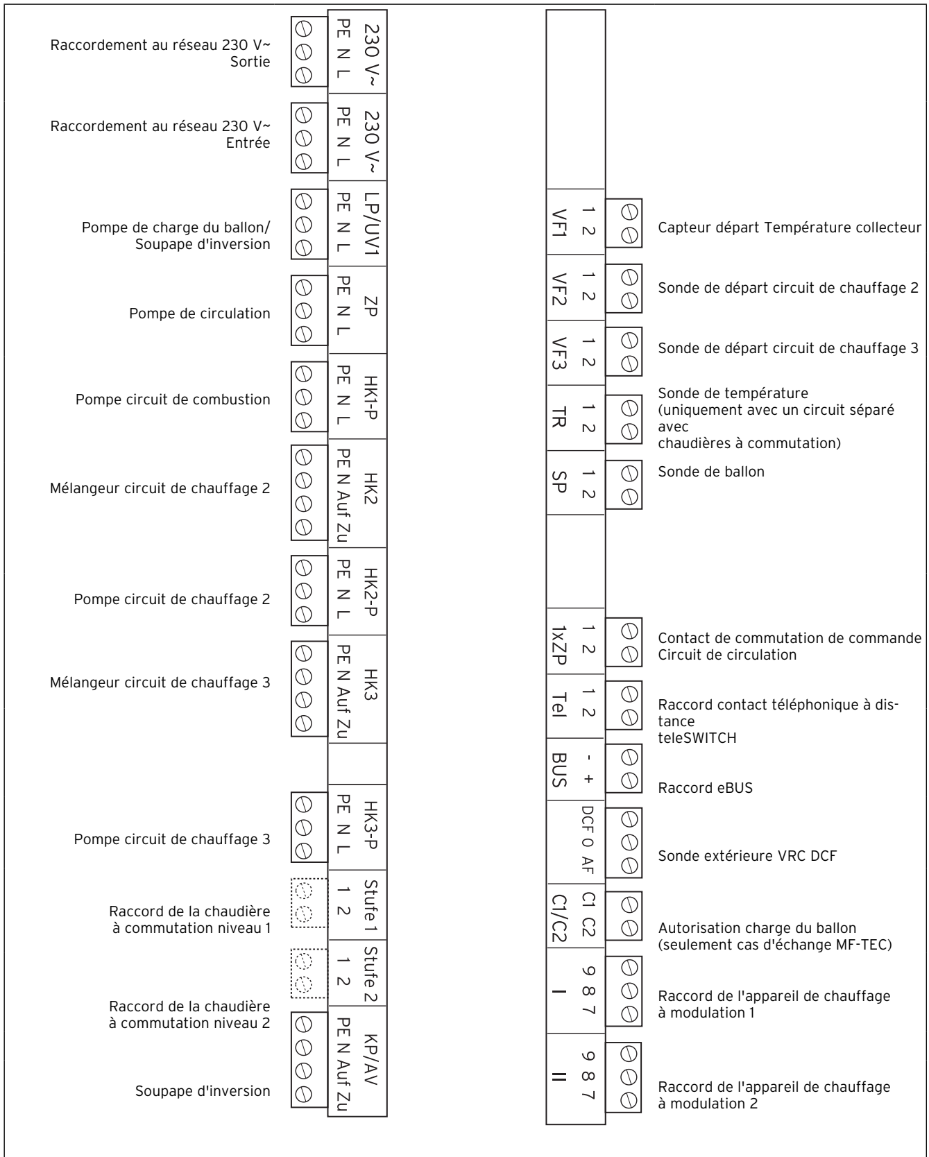
Fig. 5.4 Affectation des plots de connexion
