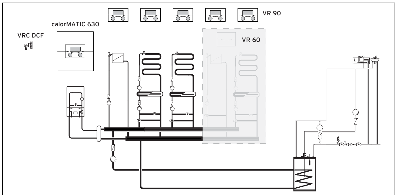
Fig. 3.1 Vue d'ensemble du système
