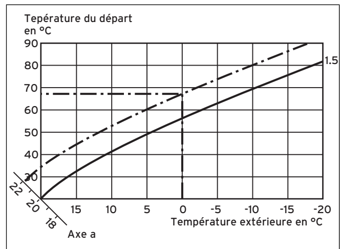
Fig. 3.4 Déplacement parallèle de la courbe de chauffage
