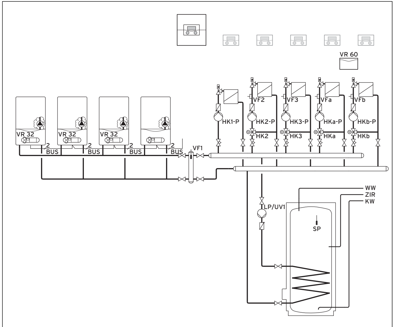
Fig. 5.6 Appareils de chauffage mural avec VRC 630 VIH derrière le compensateur
