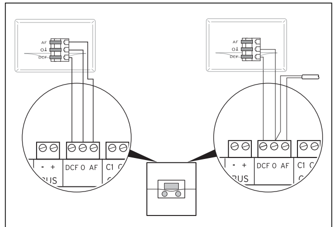
Fig.5.11 Raccord du récepteur DCF
