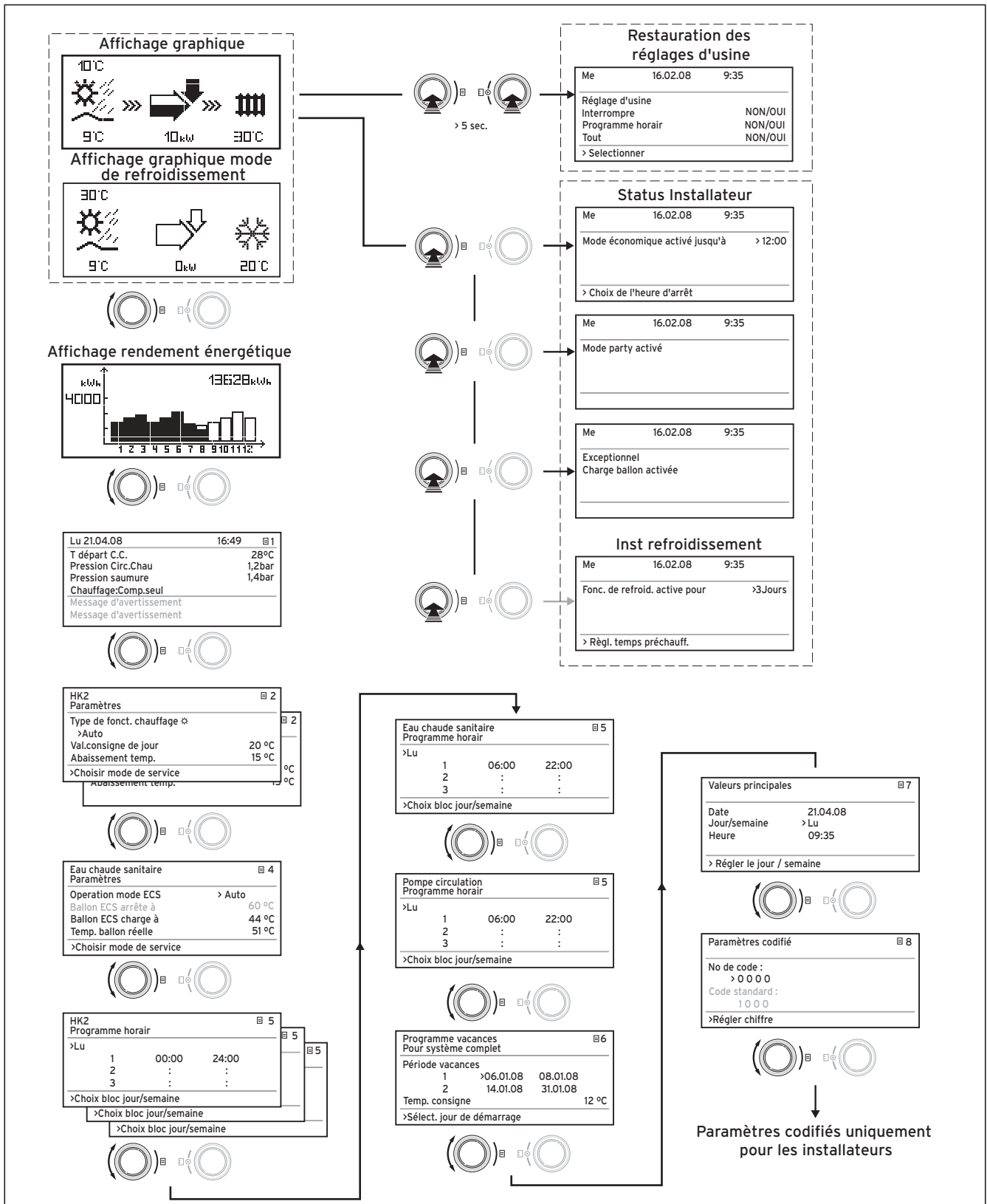
Fig. 8.1 Ecrans du niveau utilisateur
