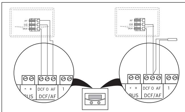
Fig. 6.11 Raccordement du récepteur DCF
