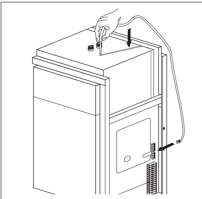
Fig. 6.7 Installation de la sonde du ballon
