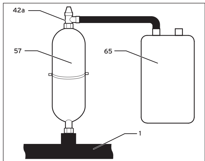
Fig. 4.13 Montage du réservoir de compensation de l'eau glycolée
