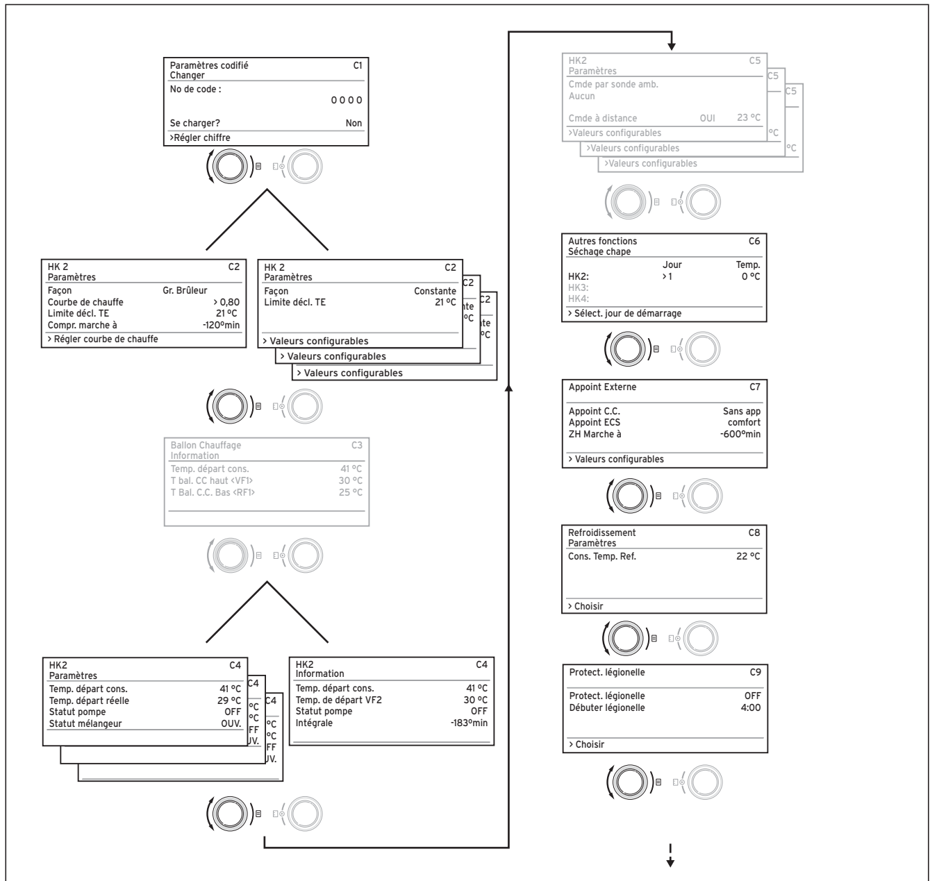
Fig. 8.2 Ecrans du niveau codé
