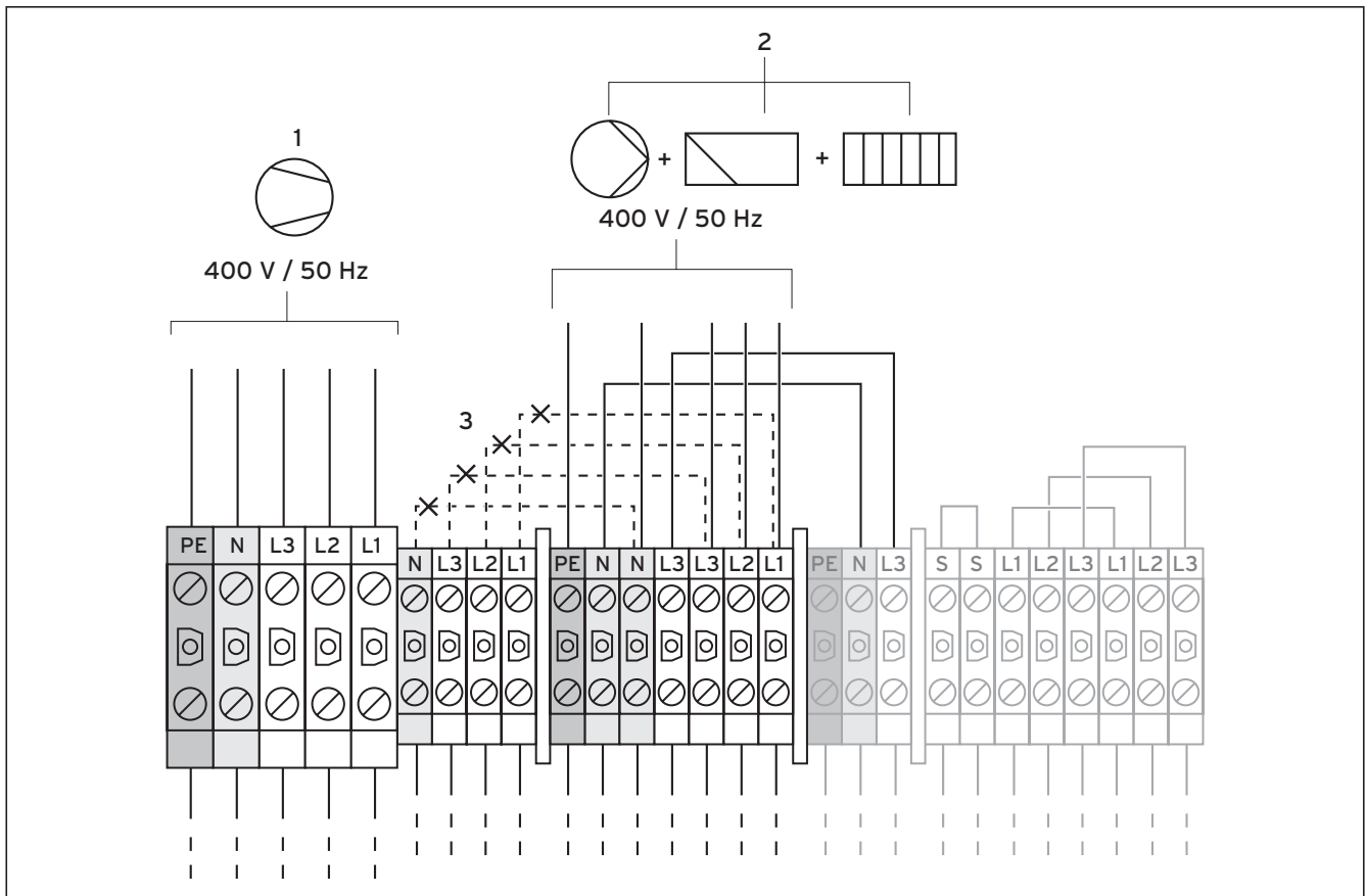
Fig. 6.3 Alimentation à deux circuits au tarif pompe à chaleur
