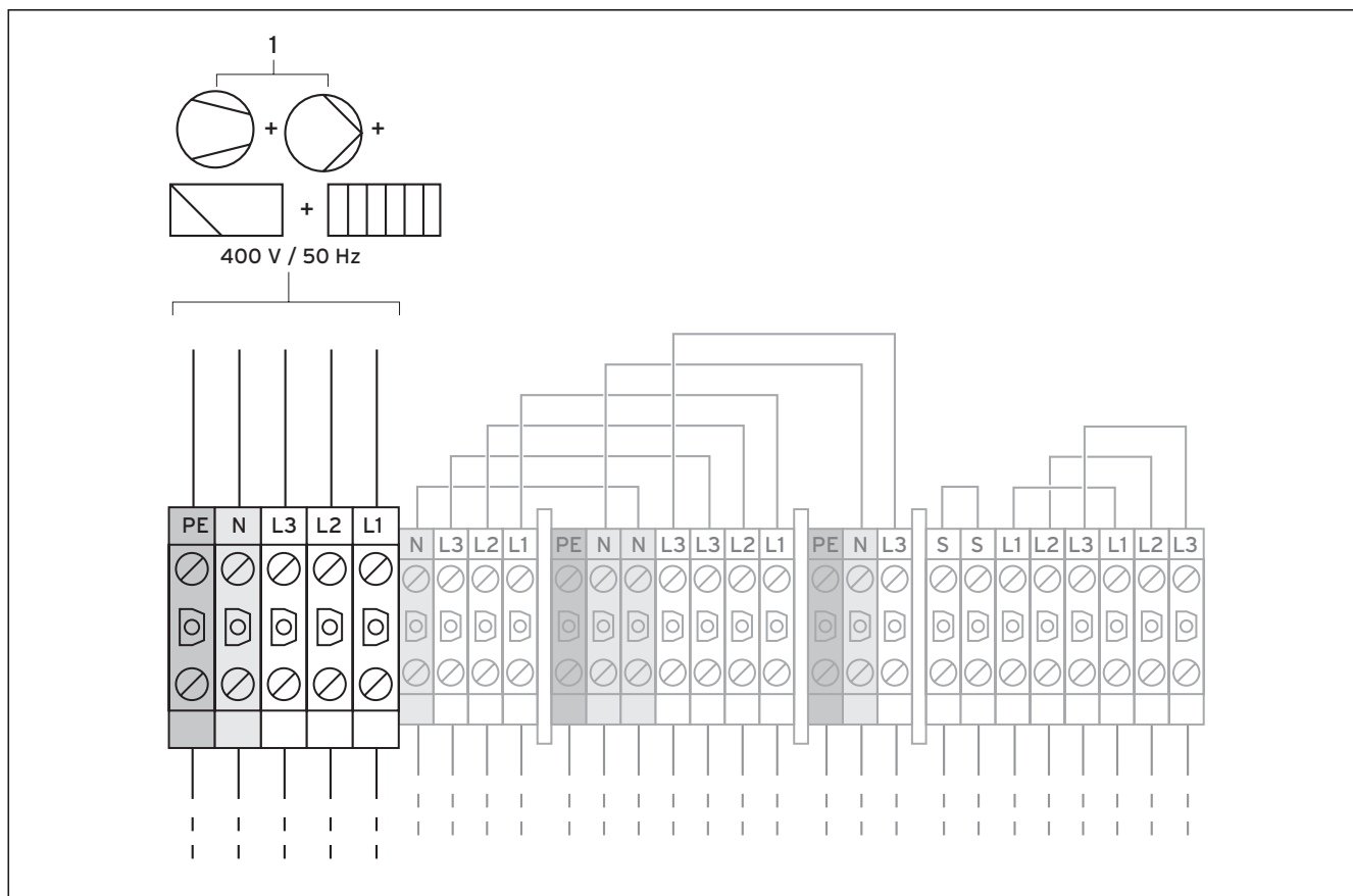
Fig. 6.2 Fourniture d'énergie au réseau non bloquée (à la livraison)
