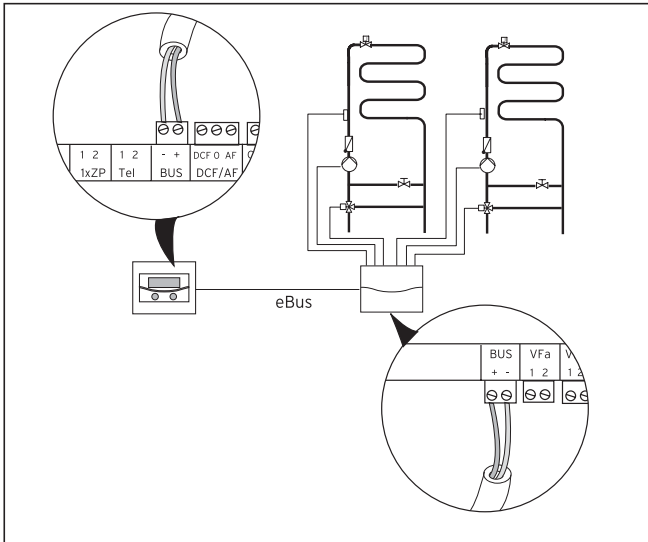
Fig. 6.14 Raccordement d'autres circuits de mélangeur
