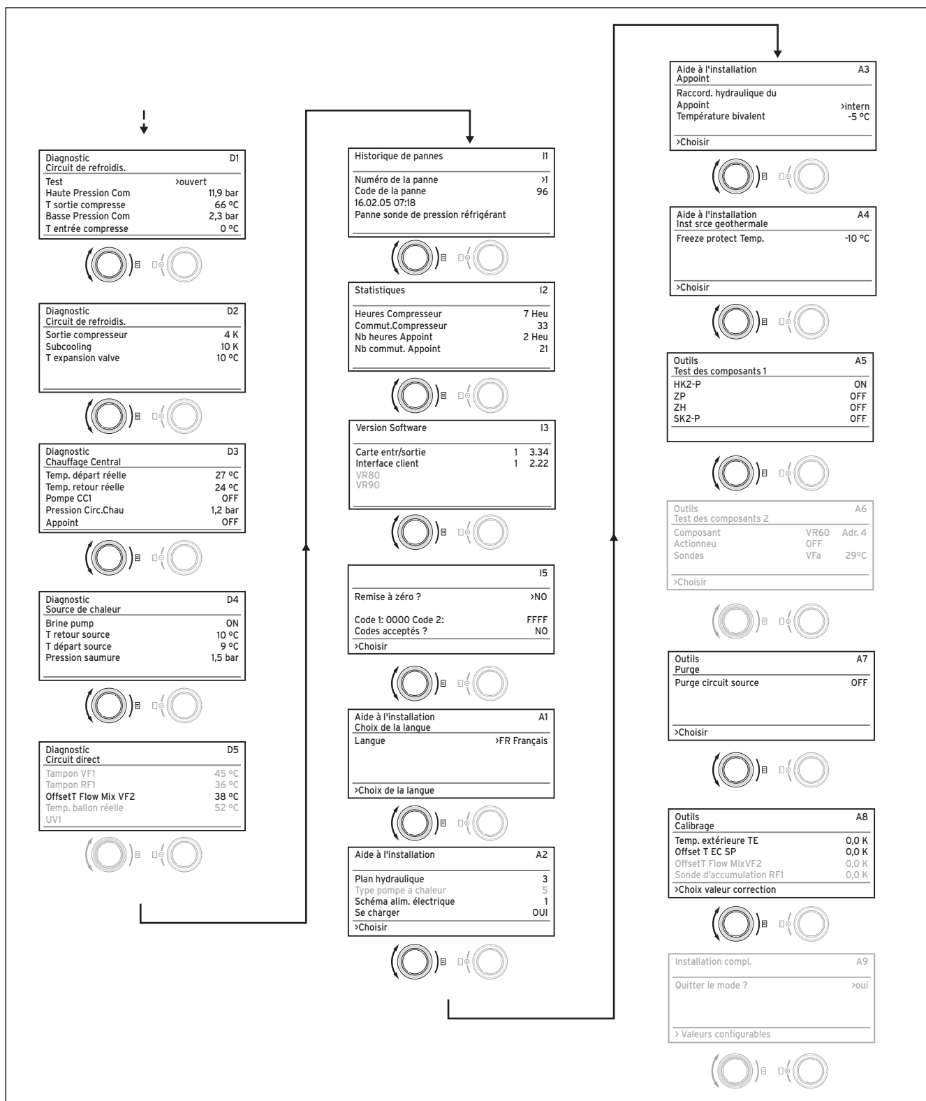
Fig. 8.3 Ecrans du niveau codé (suite)
