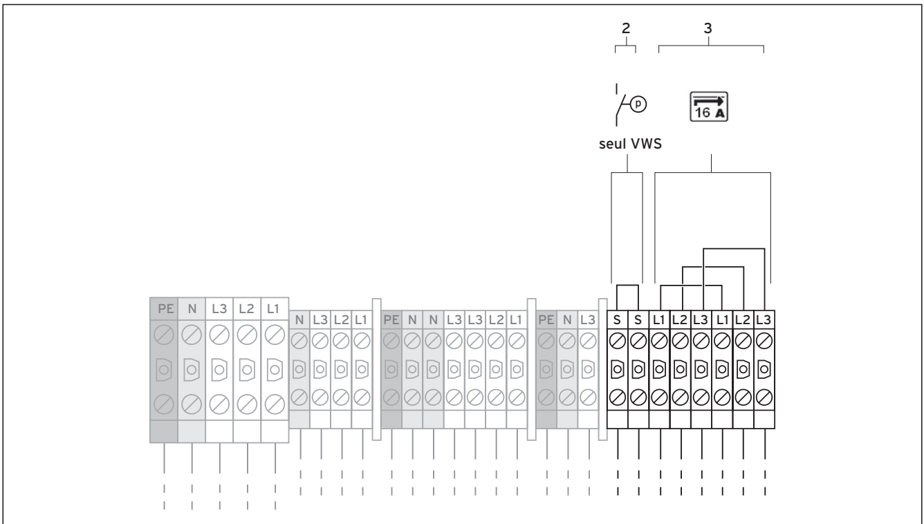
Fig. 6.5 Raccordement des composants externes
