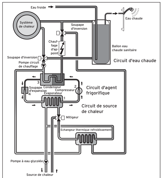
Fig. 2.3 Mode de fonctionnement de la pompe à chaleur
