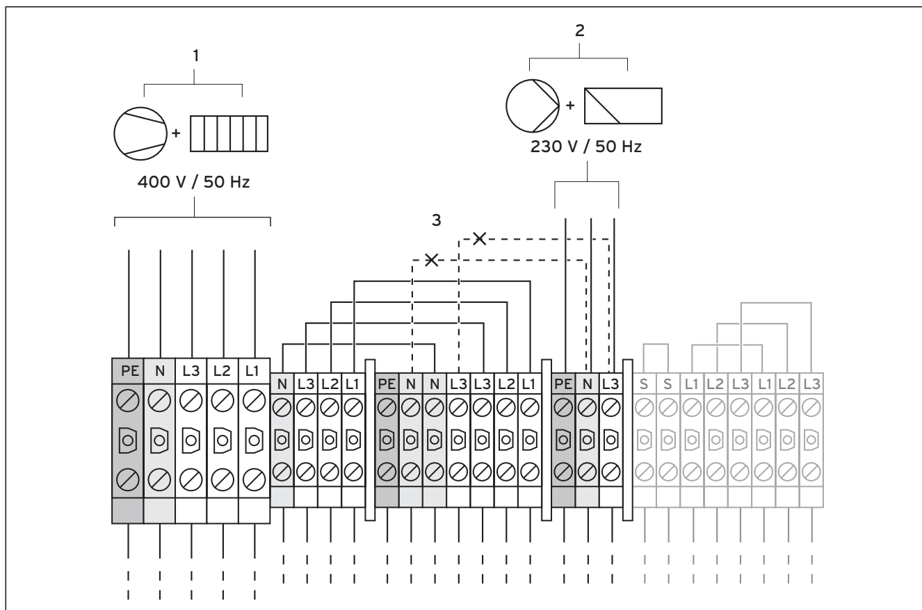
Fig. 6.4 Alimentation à deux circuits à tarif spécial
