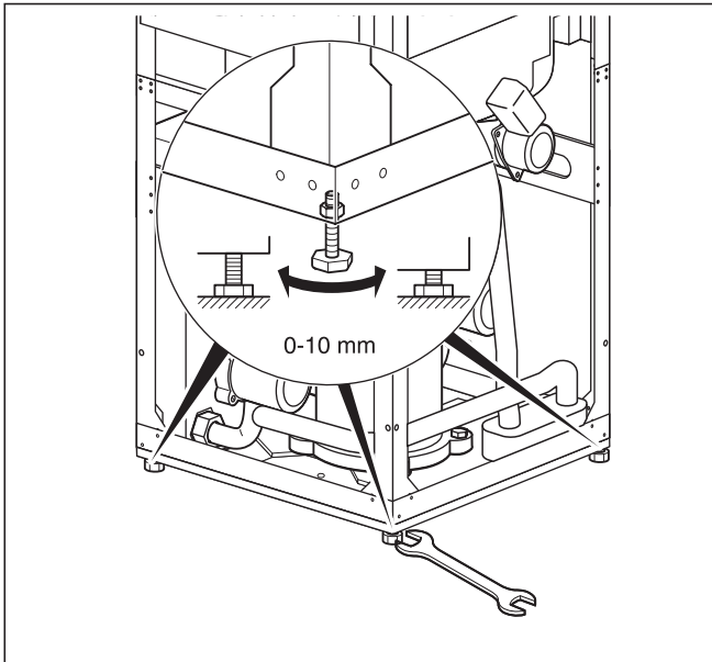
Fig. 4.10 Réglage des pieds
