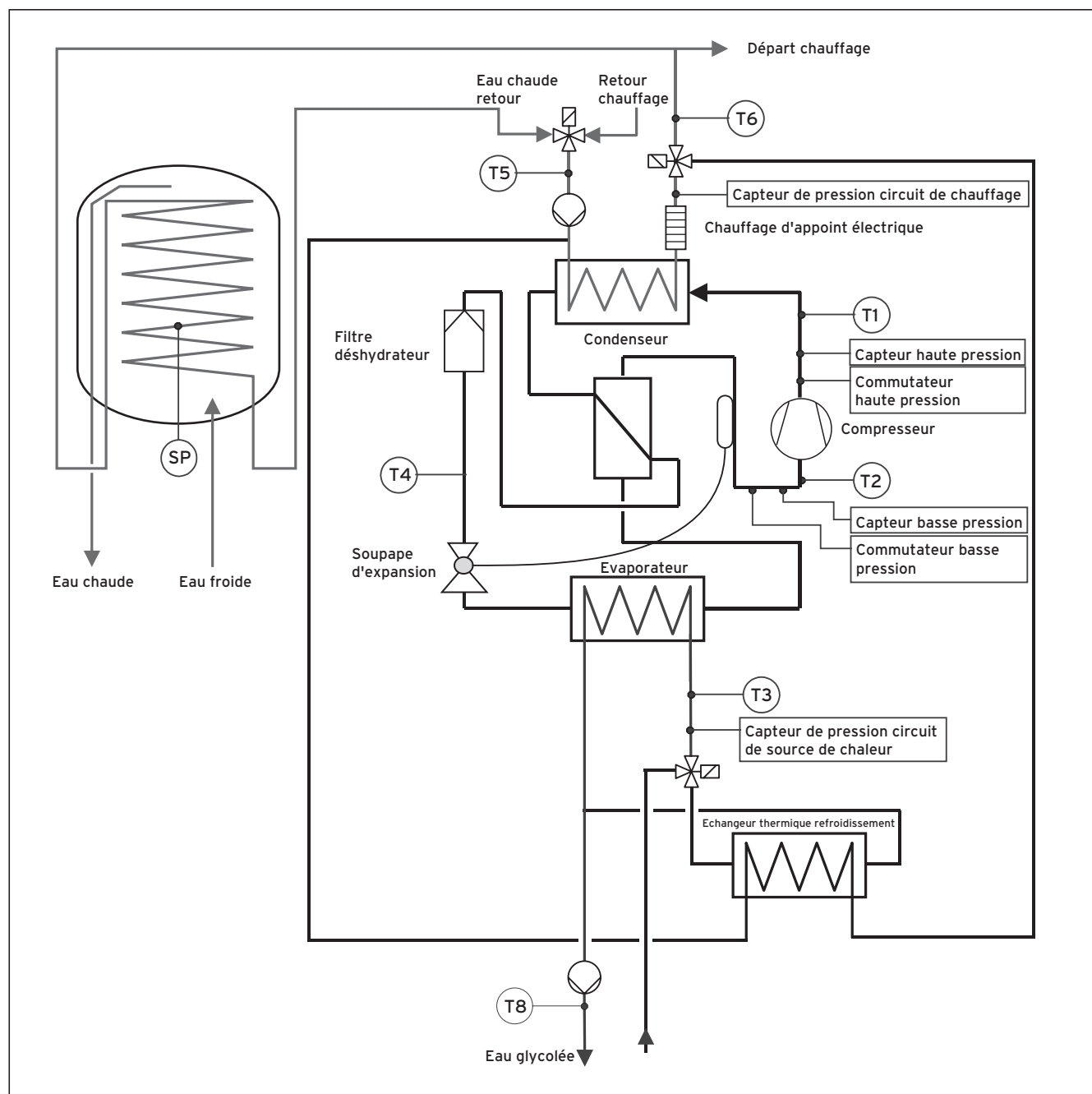
Fig. 1, Annexe, Schéma de la pompe à chaleur VWS avec ballon intégré
