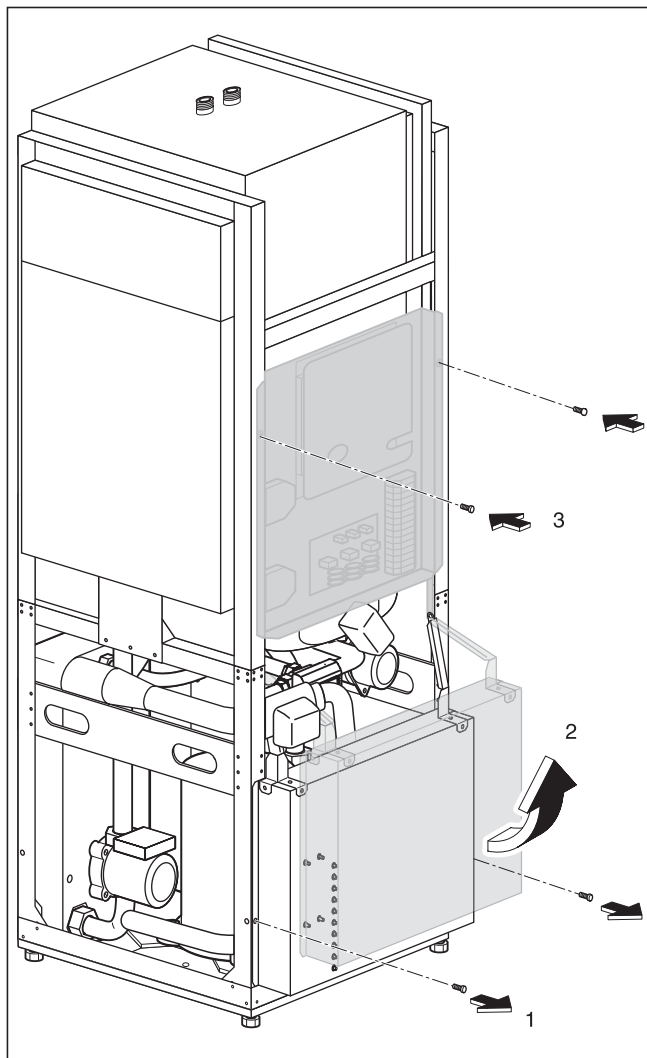
Fig. 4.9 Rabattement du boîtier de commande électrique vers le haut
