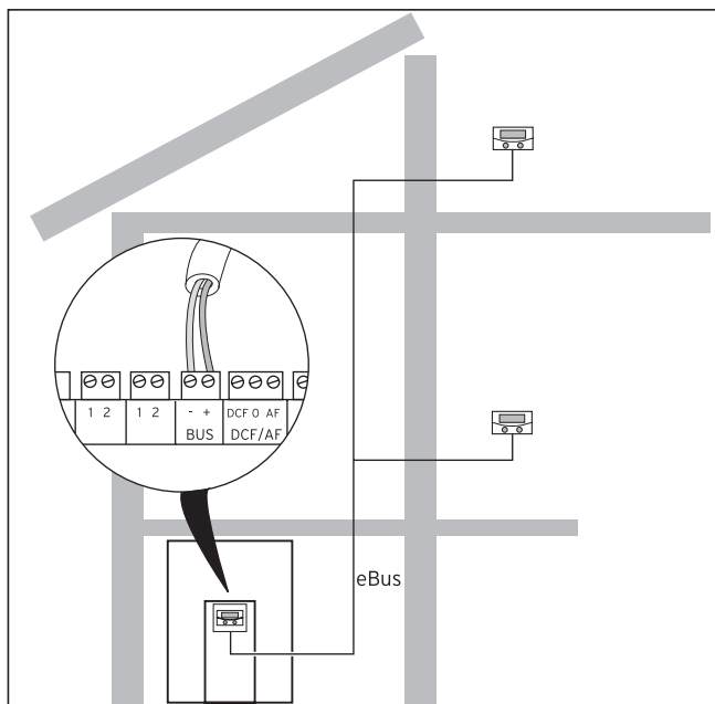
Fig. 6.12 Raccordement des télécommandes
