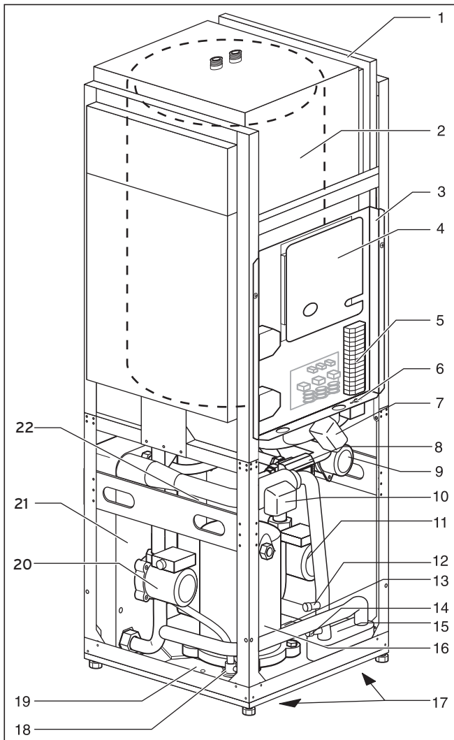
Fig. 2.7 VWS : vue avant appareil ouvert
