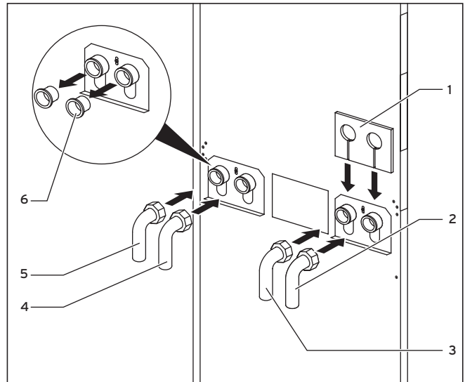
Fig. 4.11 Montage des cornières d'assemblage
