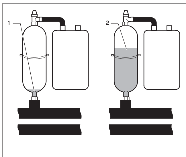
Fig. 5.8 Niveau d'eau glycolée dans le réservoir de compensation
