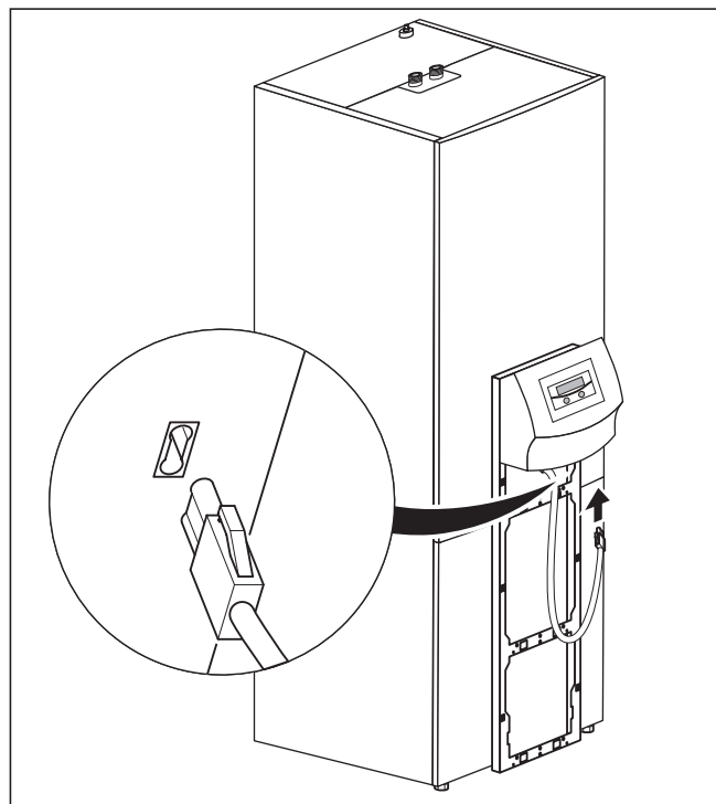
Fig. 6.24 Montage et raccordement de la console de commande
