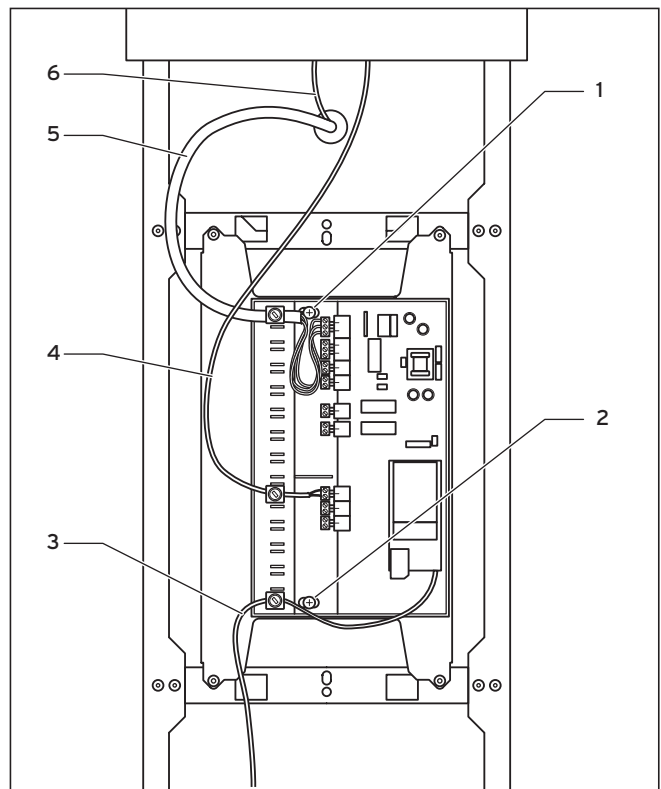
Fig. 6.16 Installation du vrnetDIALOG
