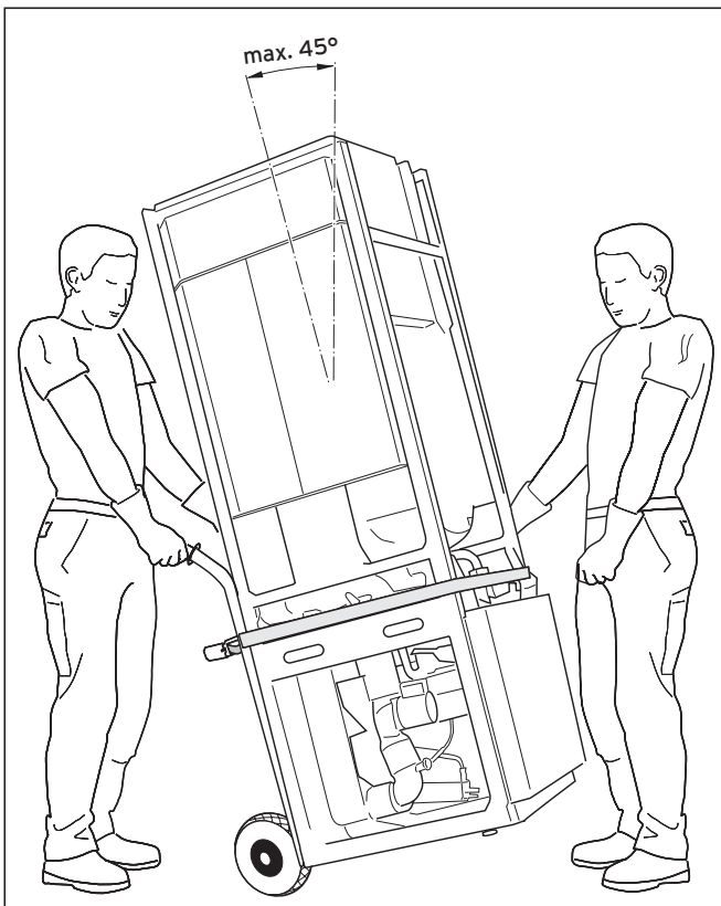
Fig. 4.7 Transport de l'installation en tant qu'unité (avec un diable)
