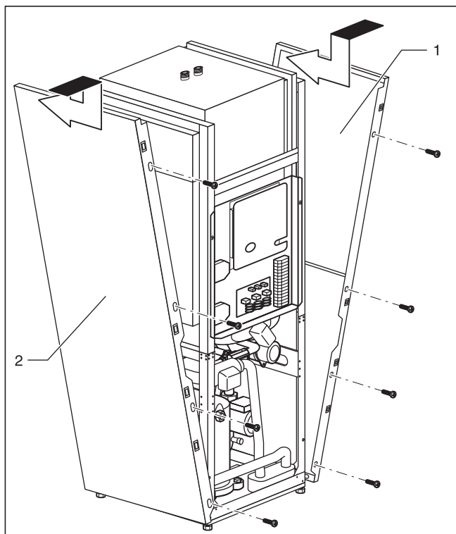
Fig. 6.19 Montage de l'habillage de protection latéral
