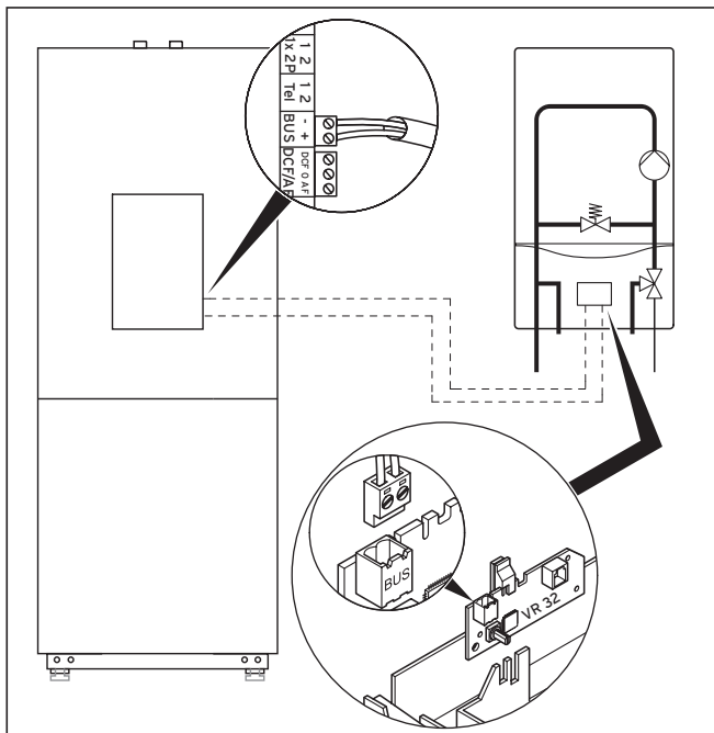
Fig. 6.17 Raccordement de l'appareil de chauffage avec interface eBus
