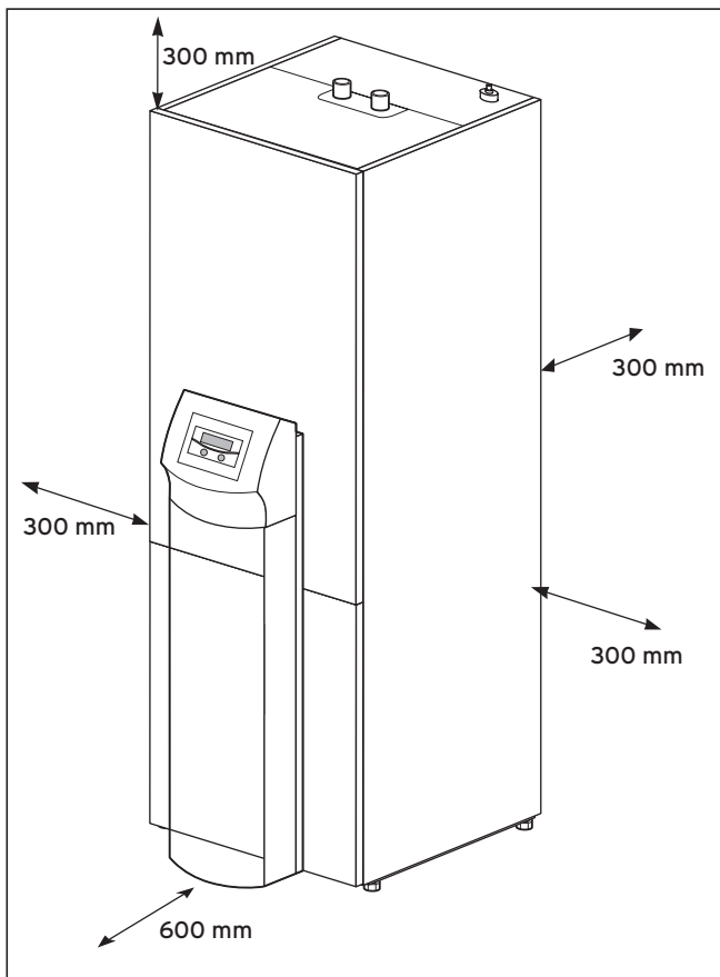
Fig. 4.2 Ecart minimum pour le montage de la pompe à chaleur
