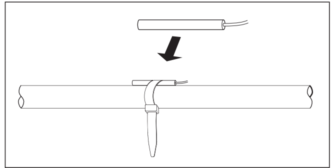
Fig. 6.7 Sonde standard VR 10
