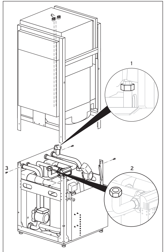
Fig. 4.8 Séparation des modules ballon d'eau potable et pompe à chaleur
