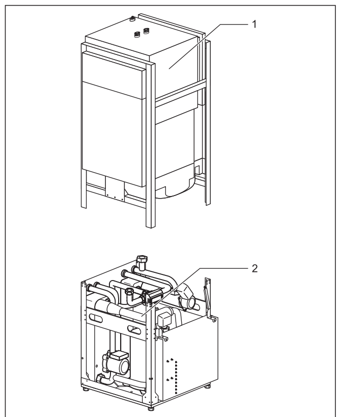
Fig. 2.4 Pompe à chaleur geoTHERM exclusiv avec modules séparables
