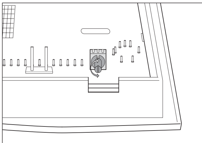
Fig. 6.13 Réglage de l'adresse bus
