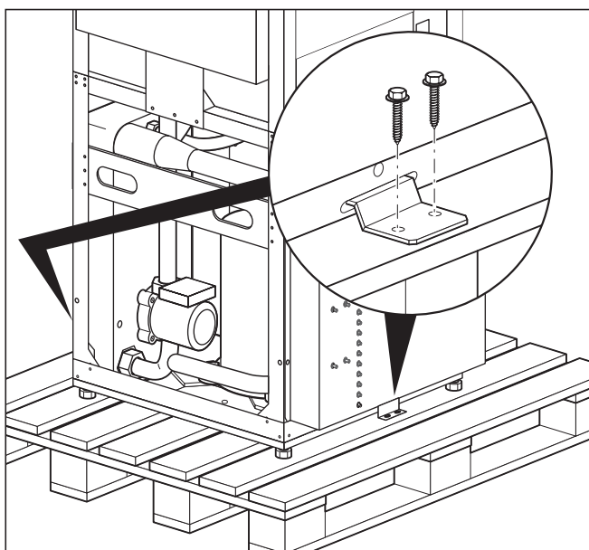
Fig. 4.5 Retrait de la protection de transport
