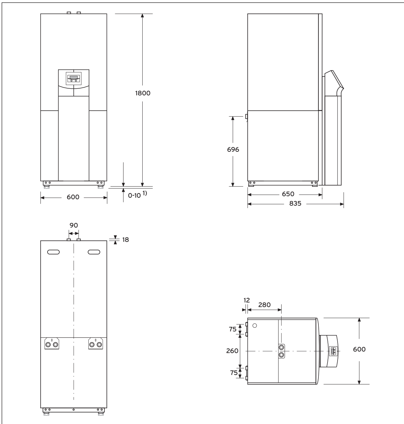
Fig. 4.1 Ecart et dimensions
