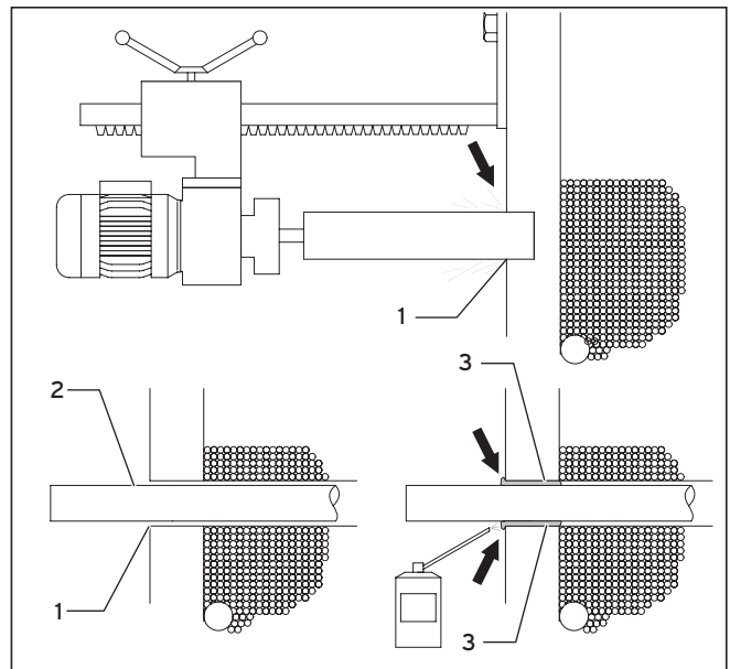
Fig. 4.3 Travaux préliminaires à effectuer sur le lieu d'installation
