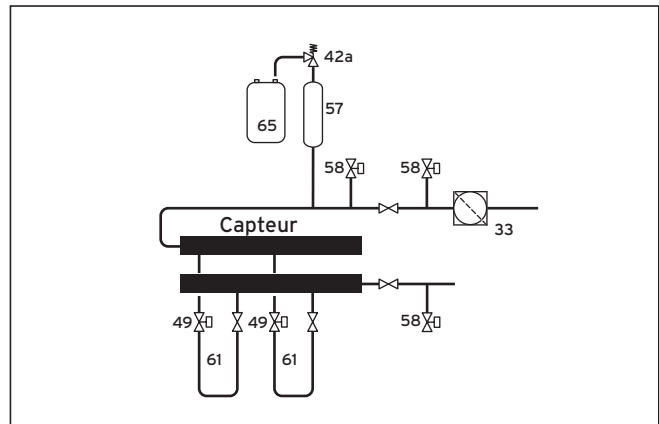
Fig. 4.12 Circuit de source de chaleur VWS
