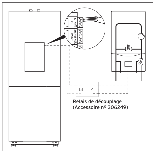
Fig. 6.18 Raccordement d'appareil de chauffage sans interface eBus
