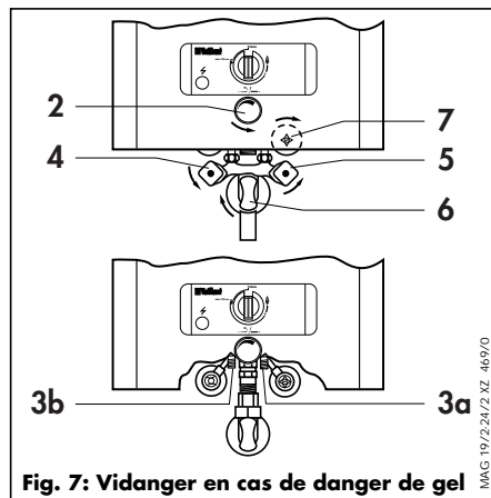
Fig. 7: Vidanger en cas de danger de gel
