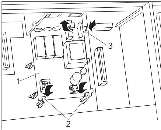
Abb. 3.1 Platine einrasten
