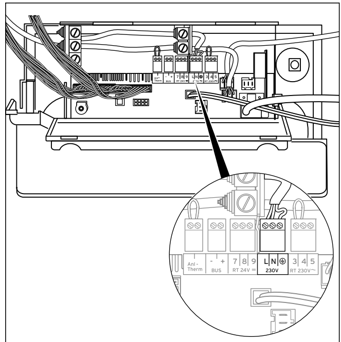
Fig. 5.11 Raccordement de l'alimentation réseau
