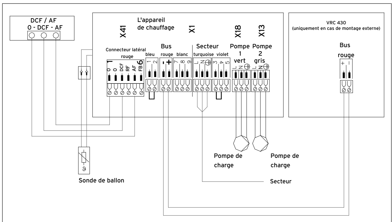
Fig. 5.14 Raccordement de l'appareil de régulation VRC 430
