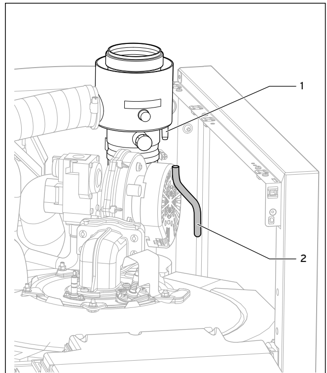
Fig. 8.3 Nettoyage du siphon
