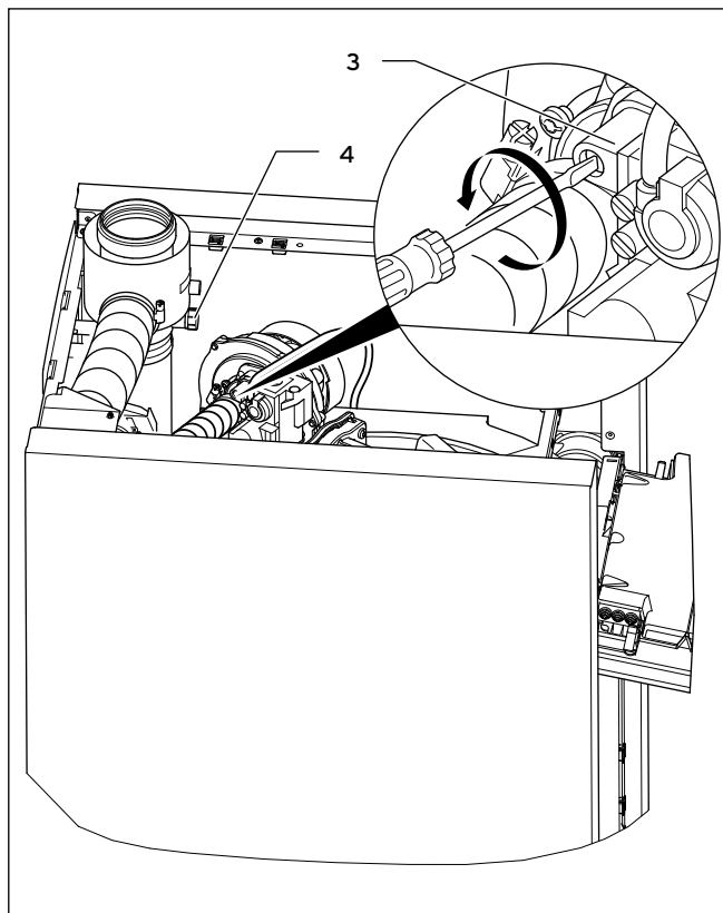
Fig. 6.4 Contrôle CO 2
