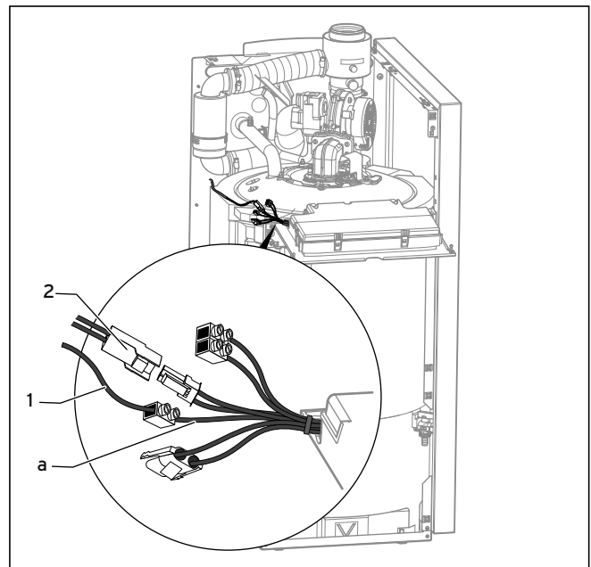
Fig. 5.5 Raccordement de la sonde de ballon et sonde de température du ballon (actoSTOR)
