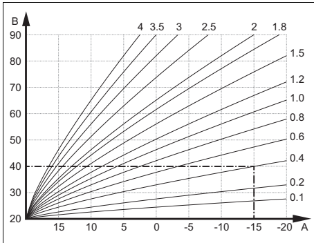
A Außentemperatur °C B Vorlauf Solltemperatur °C
