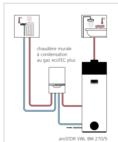
aroSTOR VWL avec si nécessaire une chauffe complémentaire via une chaudière chauffage seul
