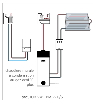
aroSTOR VWL en version "standalone" en combinaison avec des panneaux solaires thermiques et si nécessaire une chauffe complémentaire via une résistance électrique
