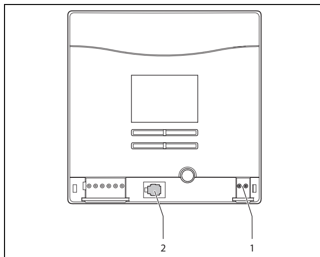
1 eBUS-aansluiting 2 Serviceaansluiting
